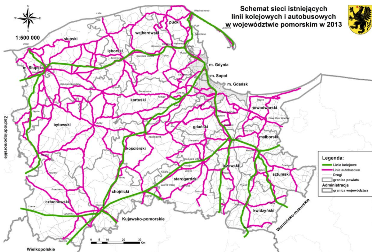
Rys. 2.5. Schemat sieci istniejących linii kolejowych i autobusowych realizujących wojewódzkie przewozy pasażerskie na obszarze województwa pomorskiego w roku 2013
